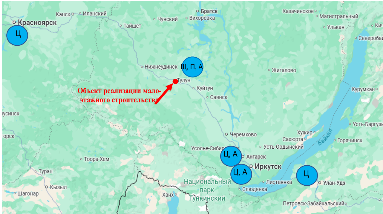
Рис. 4. Ресурсные базы для мобильного домостроительного комплекса в г. Тулун (Ц – цемент, Щ – щебень, П – песок, А – арматура)
