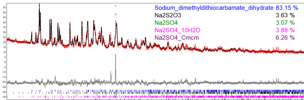
Рис. 4. Рентгенограмма образца реагента Plexon 3315 в программе TOPAS 3
