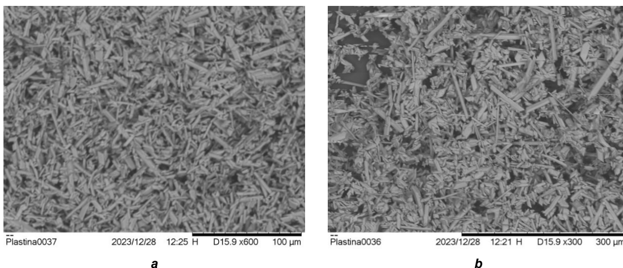
Рис. 16. Кристаллы сульфата кальция, образовавшиеся в потоке за счет пересыщения (а) и выросшие кристаллы, вымываемые из модуля (b). Степень пересыщения в потоке концентрата: 2,9
